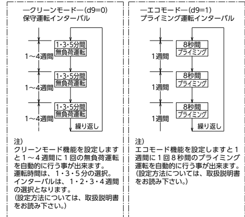
自動保守運転タイムチャート
