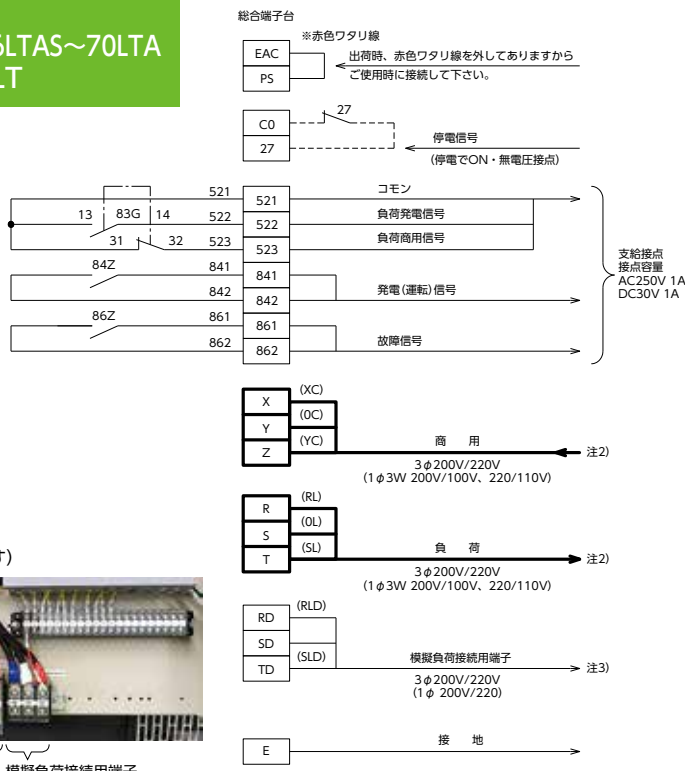
商用 負荷 模擬負荷接続用端子
